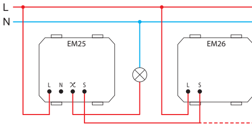
(1) 2-vezetékes bekötés two-wire connection
