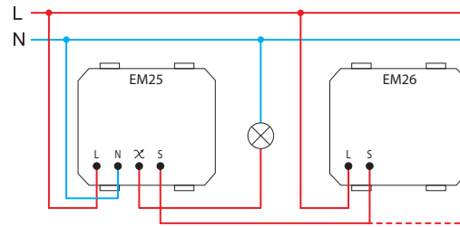
(2) 3-vezetékes bekötés three-wire connection
