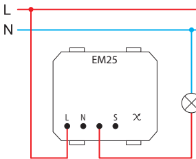
(1) 2-vezetékes bekötés two-wire connection
