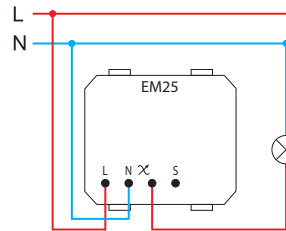
(2) 3-vezetékes bekötés three-wire connection
