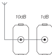
Durchgangsschaltung throughpass connection
