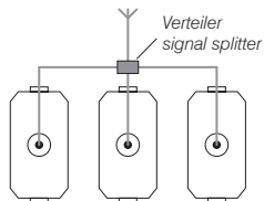
Sternschaltung star connection
