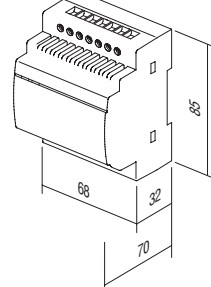
vnútorná relé jednotka interior relay unit
